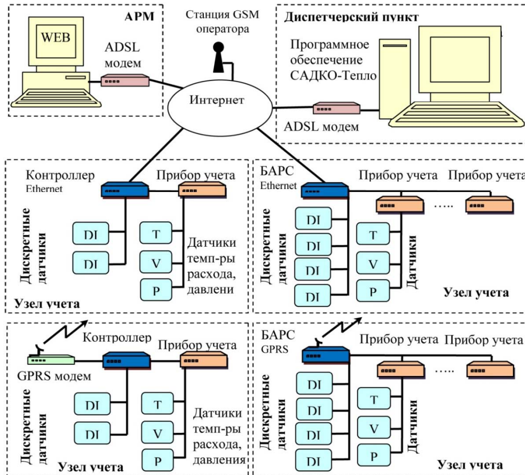
Структурная схема системы «САДКО»
